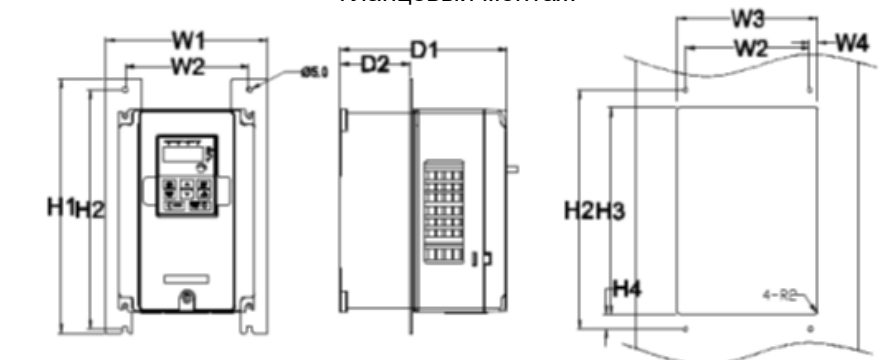
Рис. 4.12 Фланцевый монтаж 4 – 75 кВт
