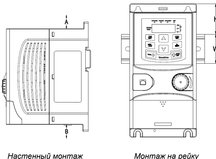
Рис. 4-1 Установка ПЧ
