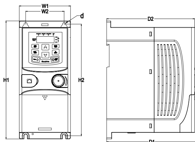
Рис. 4.7 Настенный монтаж 0.4 – 2,2 кВт
