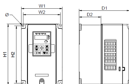
Рис. 4.9 Настенный монтаж 4 – 37 кВт
