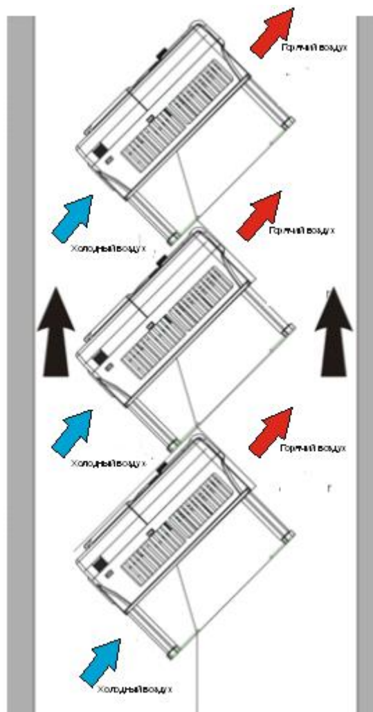
Рис. 4-6 Наклонная установка
