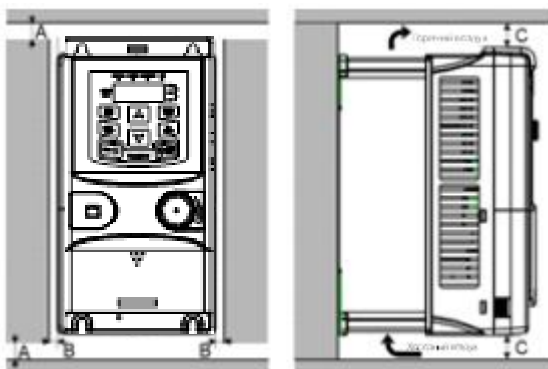
Рис. 4-3 Место установки
